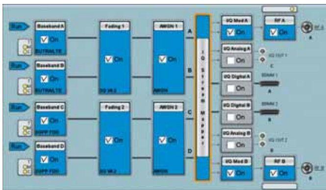
Блок-схема генератора R&S®SMW200A, настроенного на одновременную генерацию сигнала двоякой соты стандарта HSPA и 2x2 MIMO для LTE с коррелированными каналами замираний
