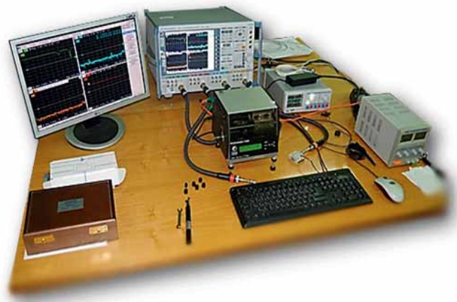
Рабочее место для измерения шумовых параметров транзисторов
